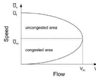
Gambar 3 Hubungan Volume dan Kecepatan
