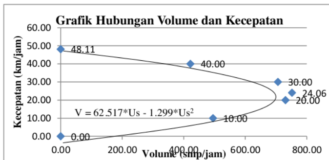
Gambar 12 Grafik Hubungan Volume dan Kecepatan Pada Hari Minggu (Hari Libur)
