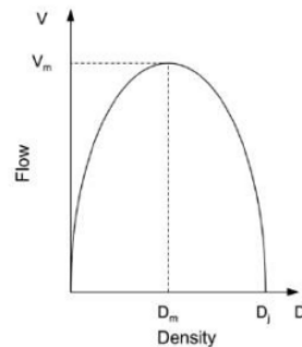
Gambar 4 Hubungan Kepadatan dan Volume
